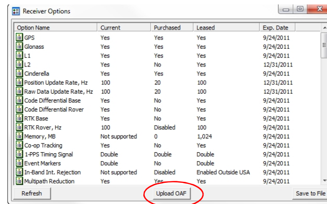
Рис. 10: Опции приемника
